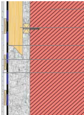
Ziegelwandaufbau
